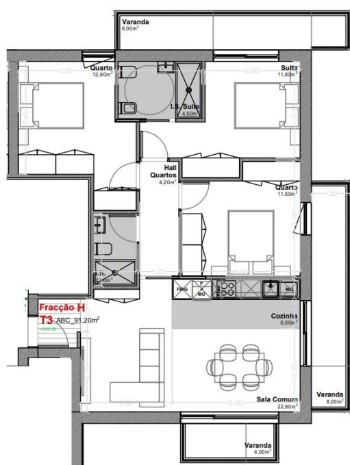
Planta da Fracção
