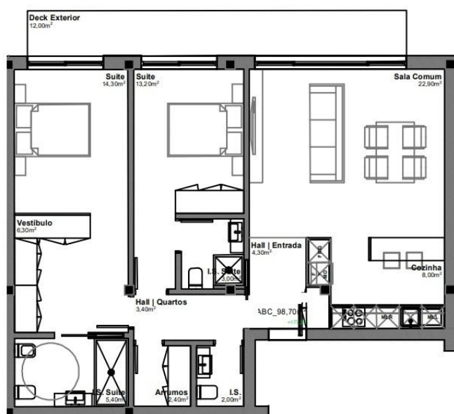
Planta da Fracção
