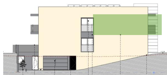
Alçado Lateral
