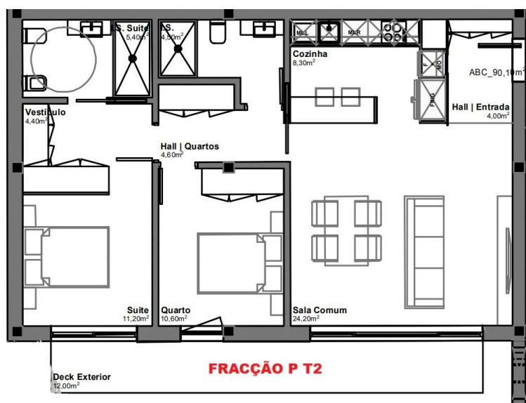
Planta da Fracção
